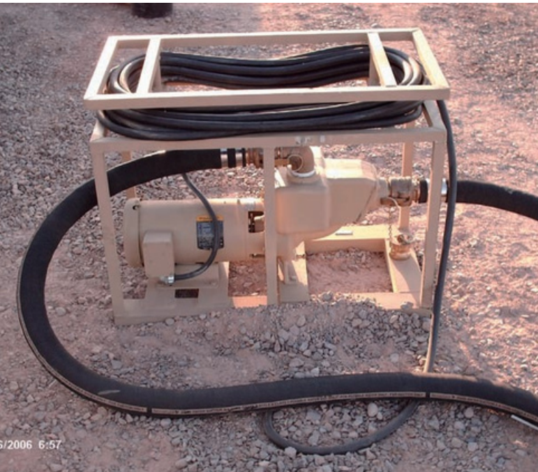
Ampco'nun RCM kendinden emişli pompası, Highland Engineering Inc'in 1500 ROWPU sistemine ham su besleme pompası olarak hizmet vermektedir
