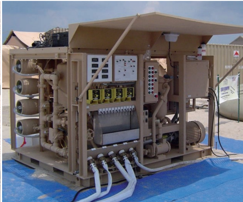
Bir Ampco ZCM pompası, son 40 yılda ABD Ordusu için binlerce tuzdan arındırma RO sisteminden birinde basıncı artırmak için kullanılıyor.
